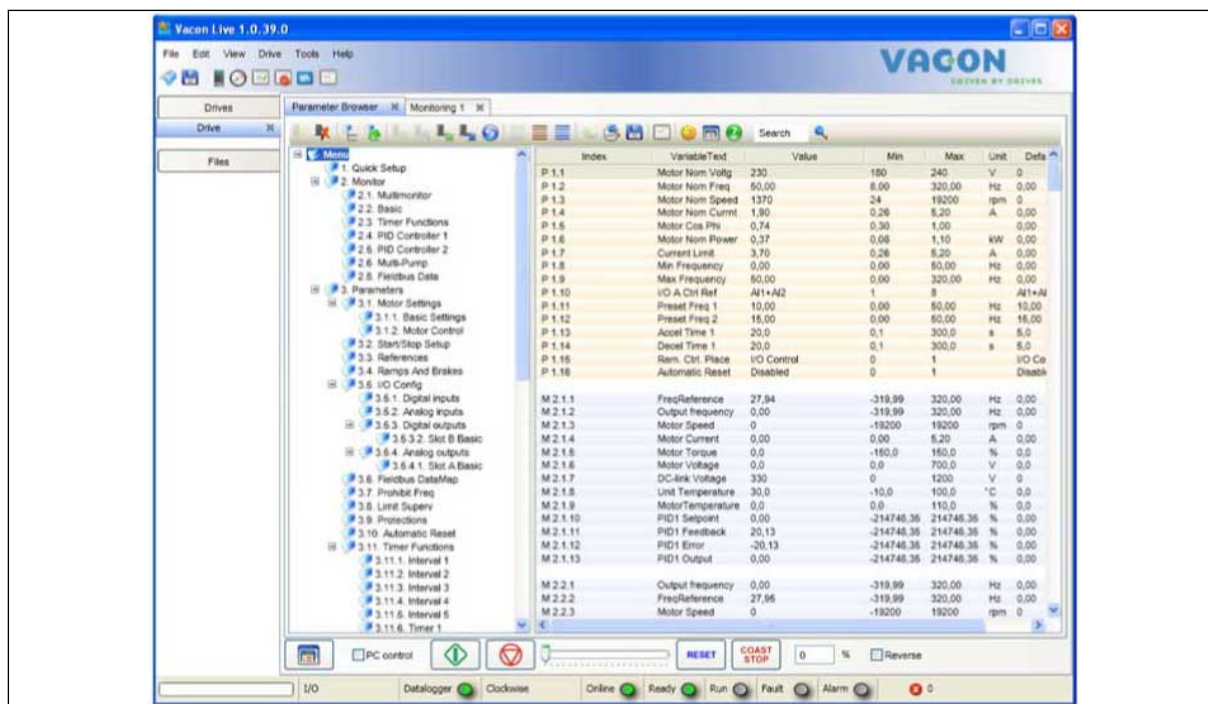
Imag. 19: La herramienta de PC Vacon Live
